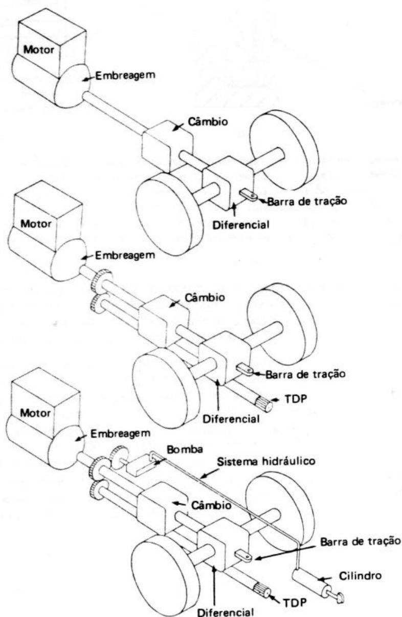
Figura 3. A evolução histórica do trator nos seus primeiros 50 anos (Mialhe, 1980)
